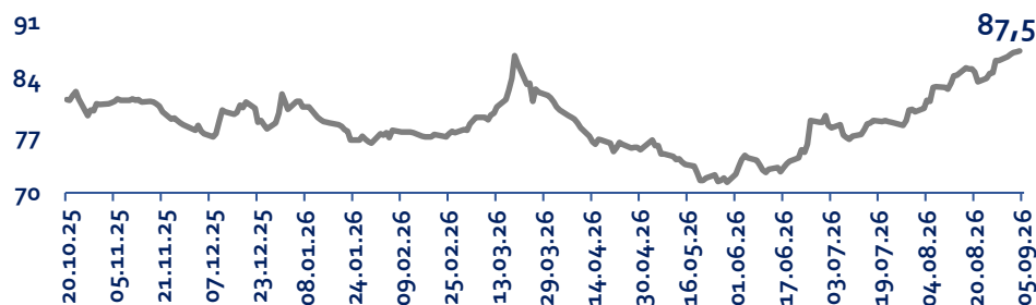
USD-RUB dinamikasi
